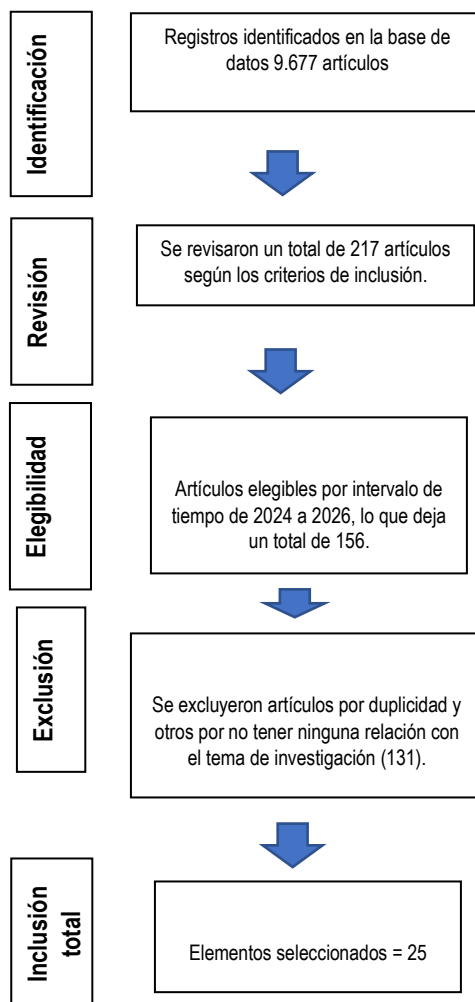
Figura 1. Flujograma PRISMA
